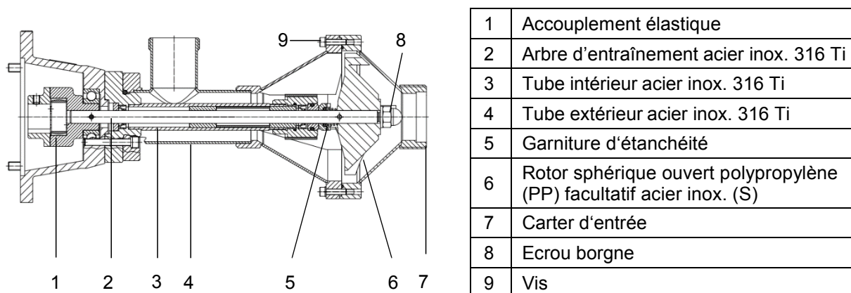
Fig. 3 Coupe de F 620 S-30 TR (exemple)
