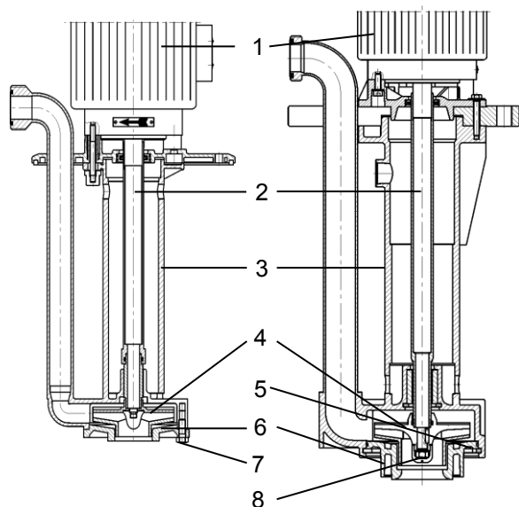
Fig. 9 Coupe de F 716 PP1-... (exemple)
