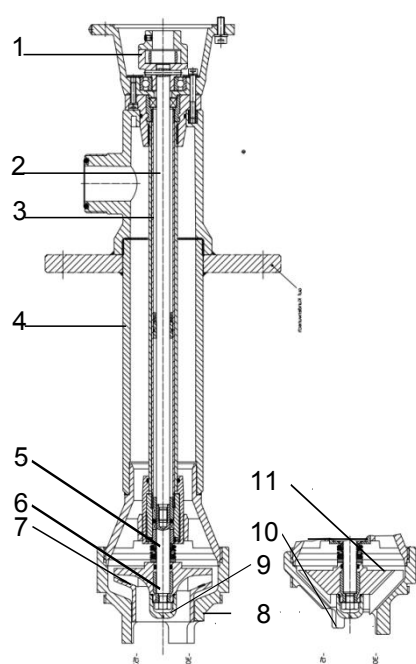
Fig. 4 Coupe de F 640 PP-15; F 640 PP-15 Z; F 640 PP-30; F 640 PP-30 Z (exemple)
