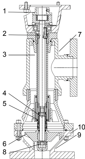
Abb. 5: Schnitt durch F 640 PP-30 TR (exemplarische Darstellung)
