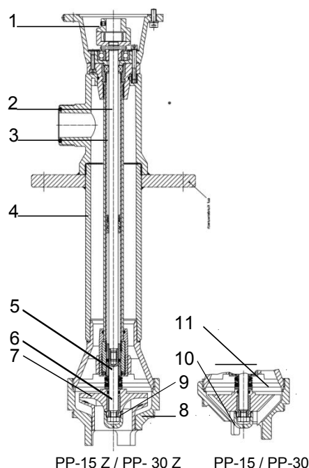
Abb. 4: Schnitt durch F 640 PP-15; F 640 PP-15 Z; F 640 PP-30; F 640 PP-30 Z (exemplarische Darstellung)
