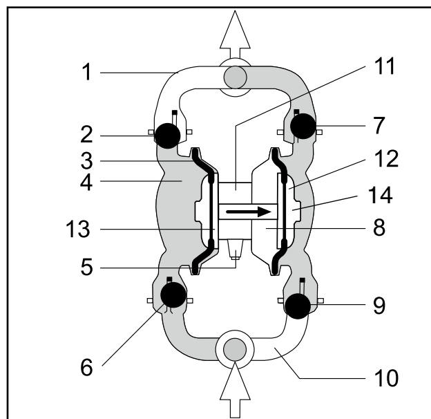
Fig. 2: Estructura de la bomba
