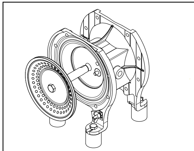
Fig. 21: Extracción del diafragma con la varilla
